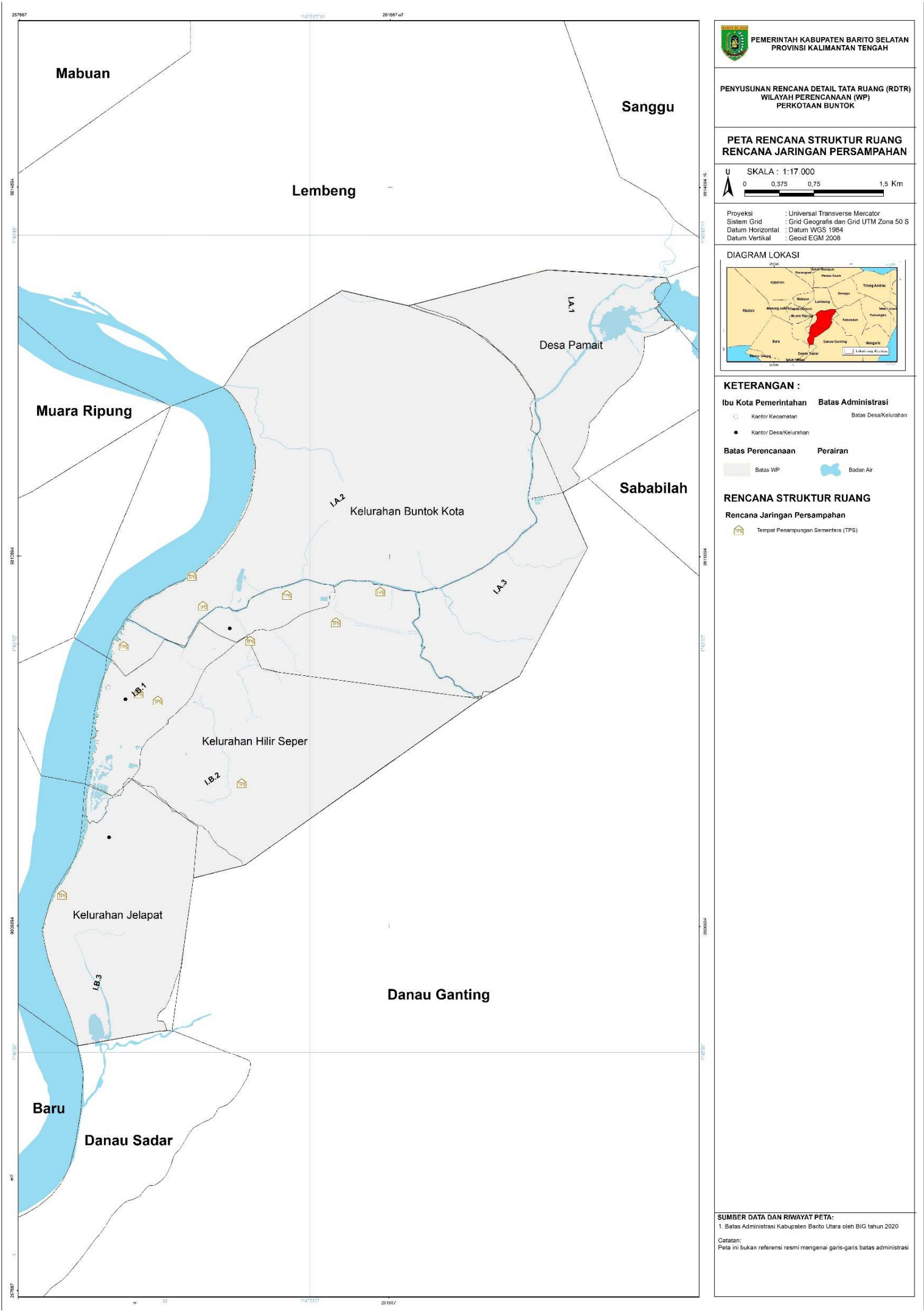
PETA RENCANA JARINGAN PERSAMPAHAN
